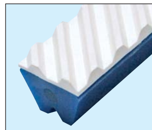
Fischgrät Beschichtung PVC weiß ca. 60° Shore A (FDA)
