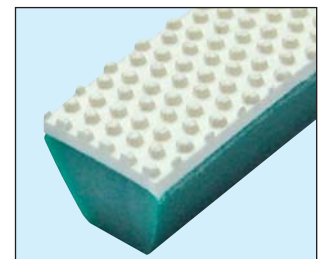
Noppen Beschichtung PVC weiß 40° Shore A (FDA)
